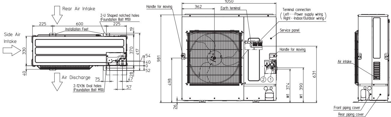
Urządzenia zewnętrzne Standard Inverter, PUHZ-P100/125/140VKA/YKA
