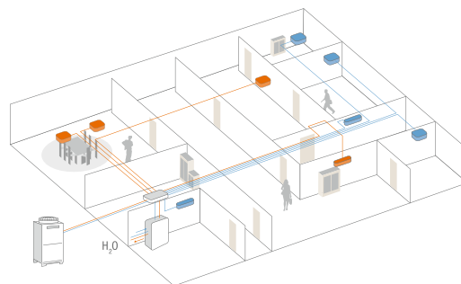
Zasada działania ekonomicznego systemu 2-rurowego z odzyskiem ciepła do jednoczesnego chłodzenia i ogrzewania.
