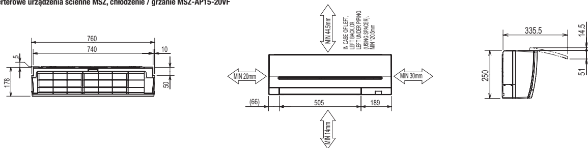
Inwerterowe urządzenia ściennie MSZ, chłodzenie / grzanie MSZ-AP15-20VF
