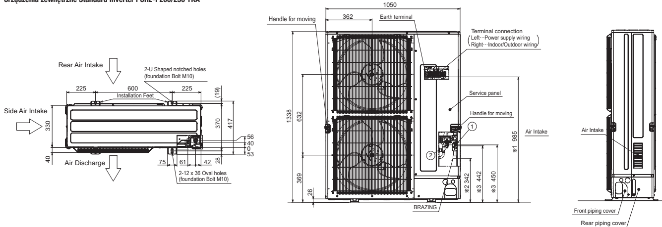
Urządzenia zewnętrzne Standard Inverter PUHZ-P200/250 YKA
