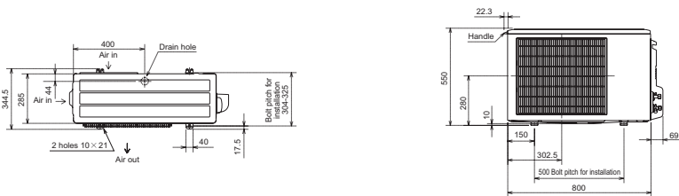
Inwerterowe urządzenia zewnętrzne MUZ, chłodzenie / grzanie MUZ-EF25-42VE
