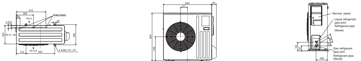
Inwerterowe urządzenia zewnętrzne MUZ, chłodzenie / grzanie MUZ-EF50VE
