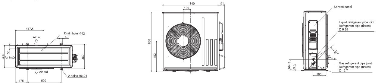
Inwerterowe urządzenia zewnętrzne MUZ, chłodzenie / grzanie MUZ-LN50-60VG(HZ)
